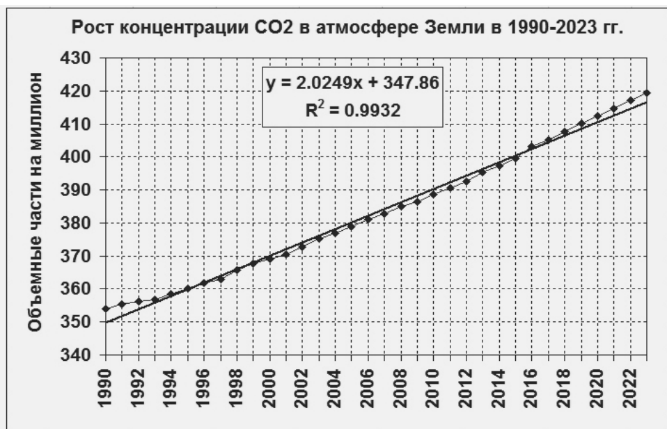
Рис. 13. Ход концентрации \text{CO}_2 в атмосфере по данным измерений в 1990–2023 гг.
