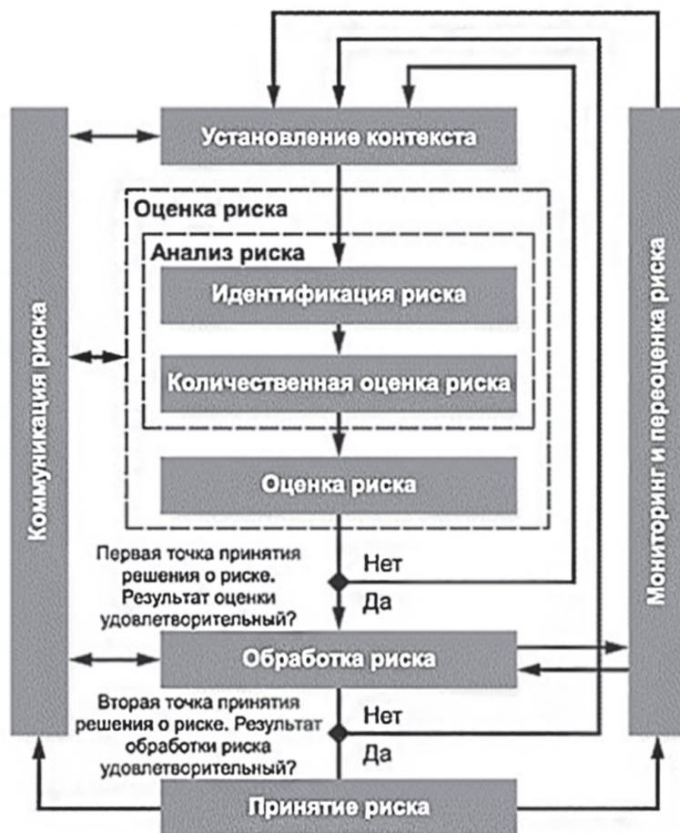
Рисунок 1. Процесс менеджмента риска информационной безопасности
