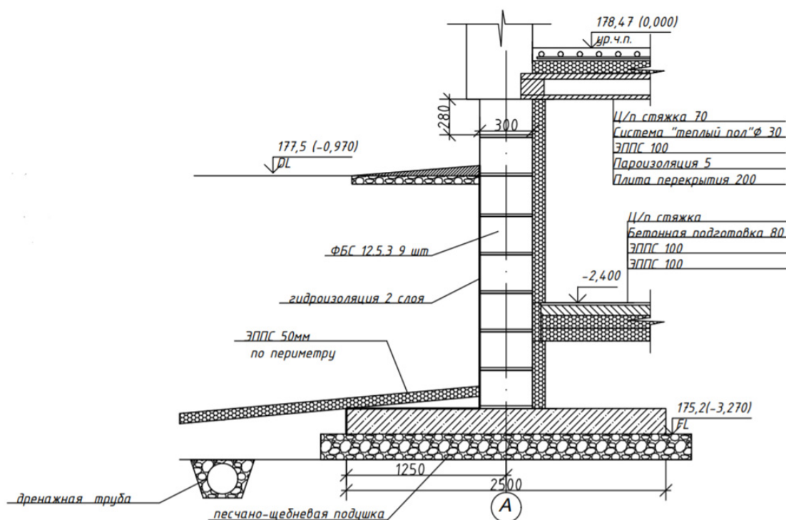
Рисунок 5. Схема утепленного финского фундамента
