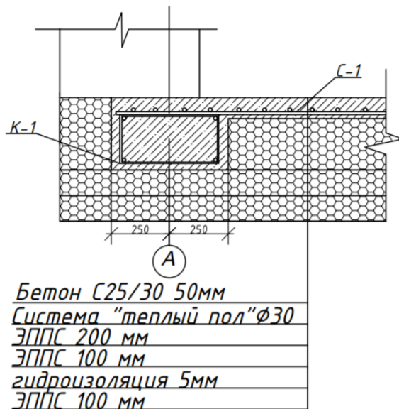
Рисунок 4. Схема утепленной шведской плиты
