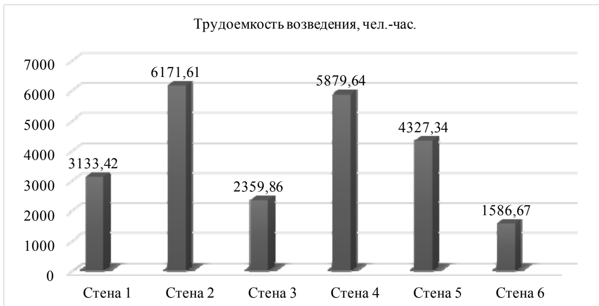
Рисунок 3. Трудоемкость возведения по вариантам проектирования
