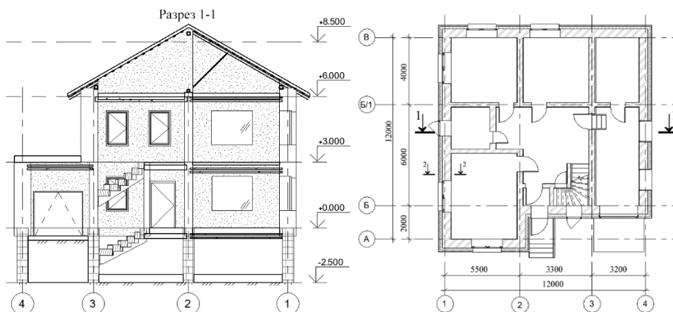
Рисунок 1. Схема здания
