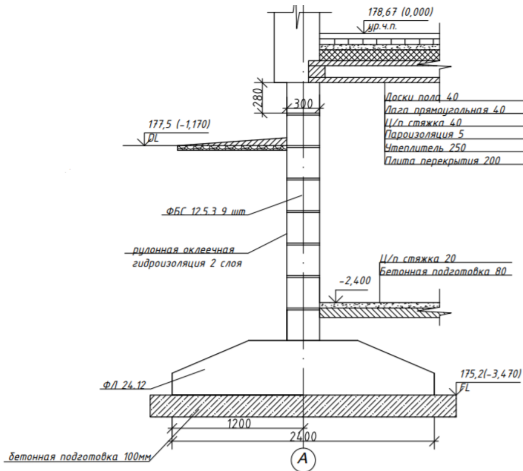
Рисунок 6. Схема ленточного фундамента
