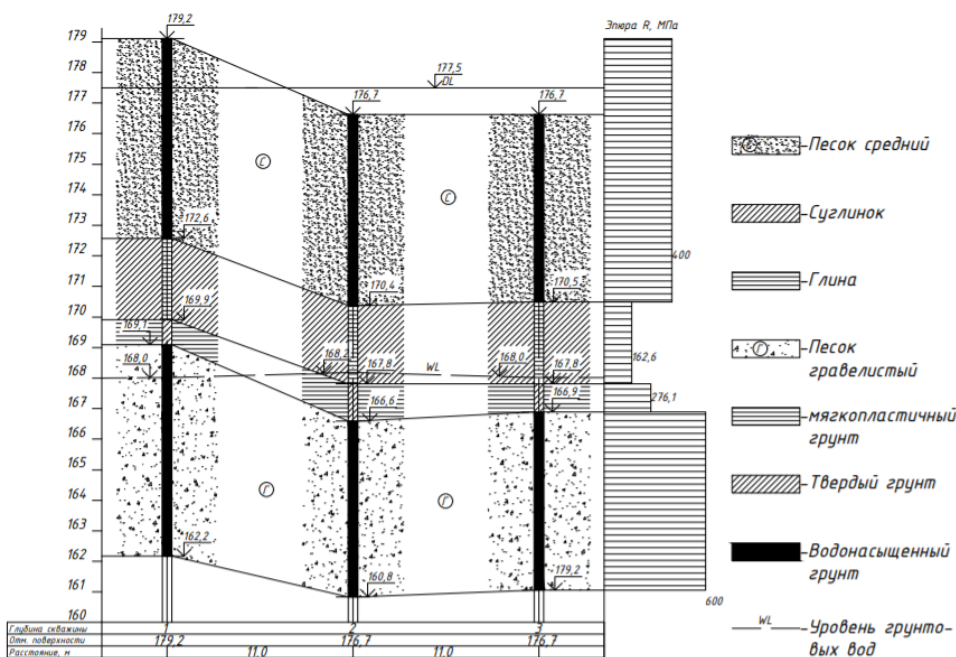
Рисунок 3. Инженерно-геологический разрез
