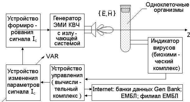
Рис. 10. Общая блок-схема эксперимента по инициации вирусоизлучения
