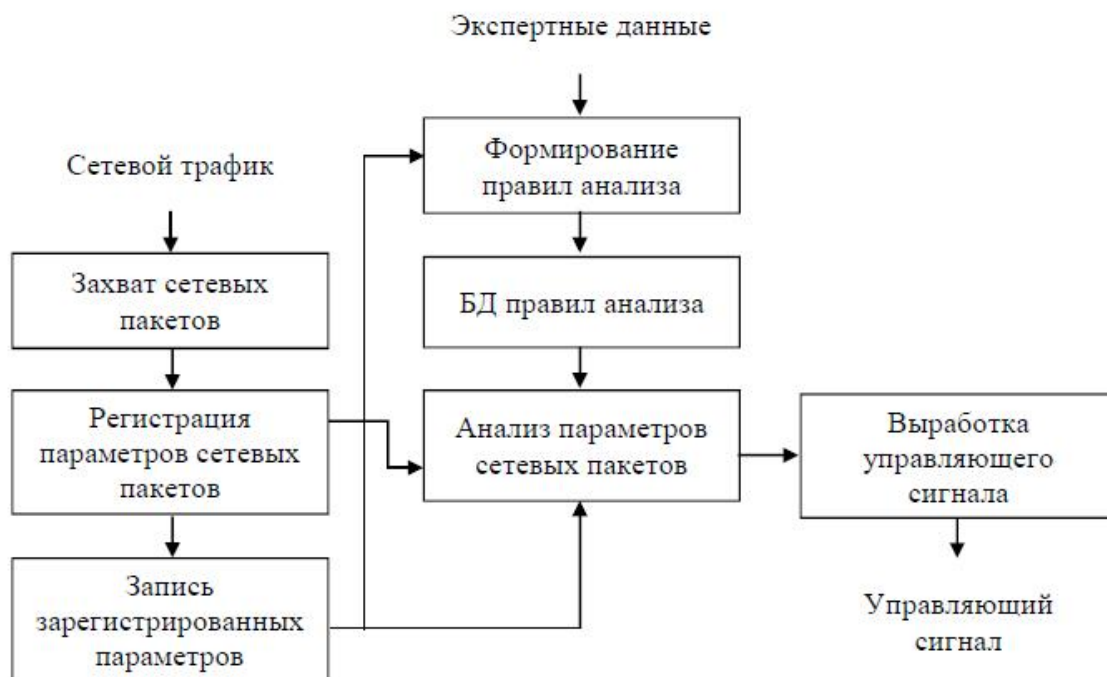
Рис. 1. Типовая последовательность функционирования сетевой СПА
